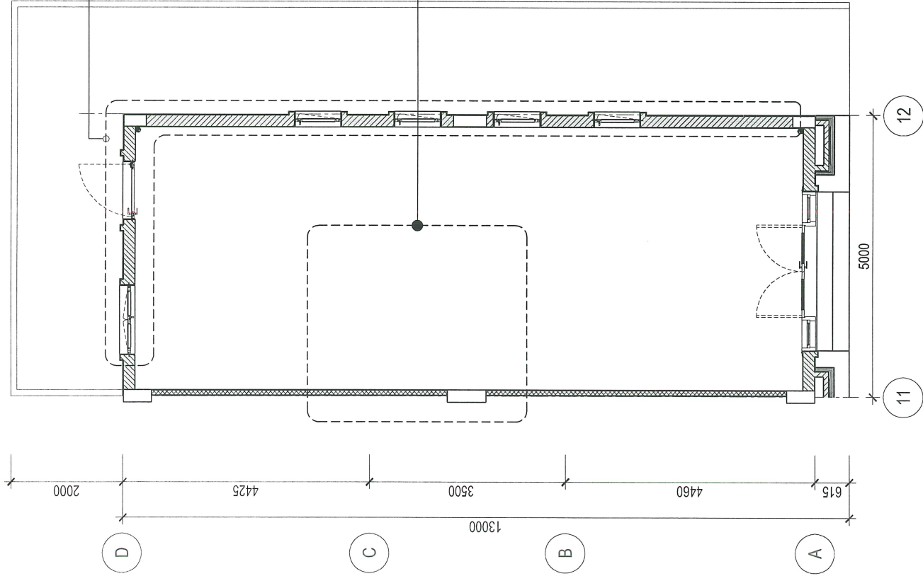
MẶT BẰNG HIỆN TRẠNG TẦNG 1
