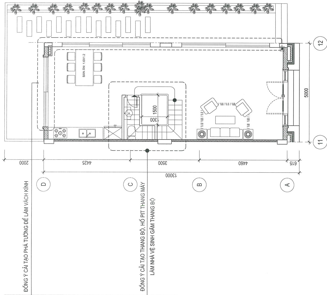
MẶT BẰNG CẢI TẠO TẦNG 1
