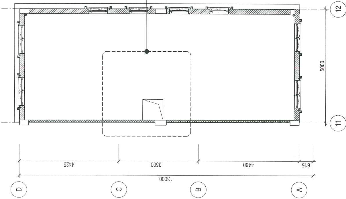
MẶT BẰNG HIỆN TRẠNG TẦNG 3
