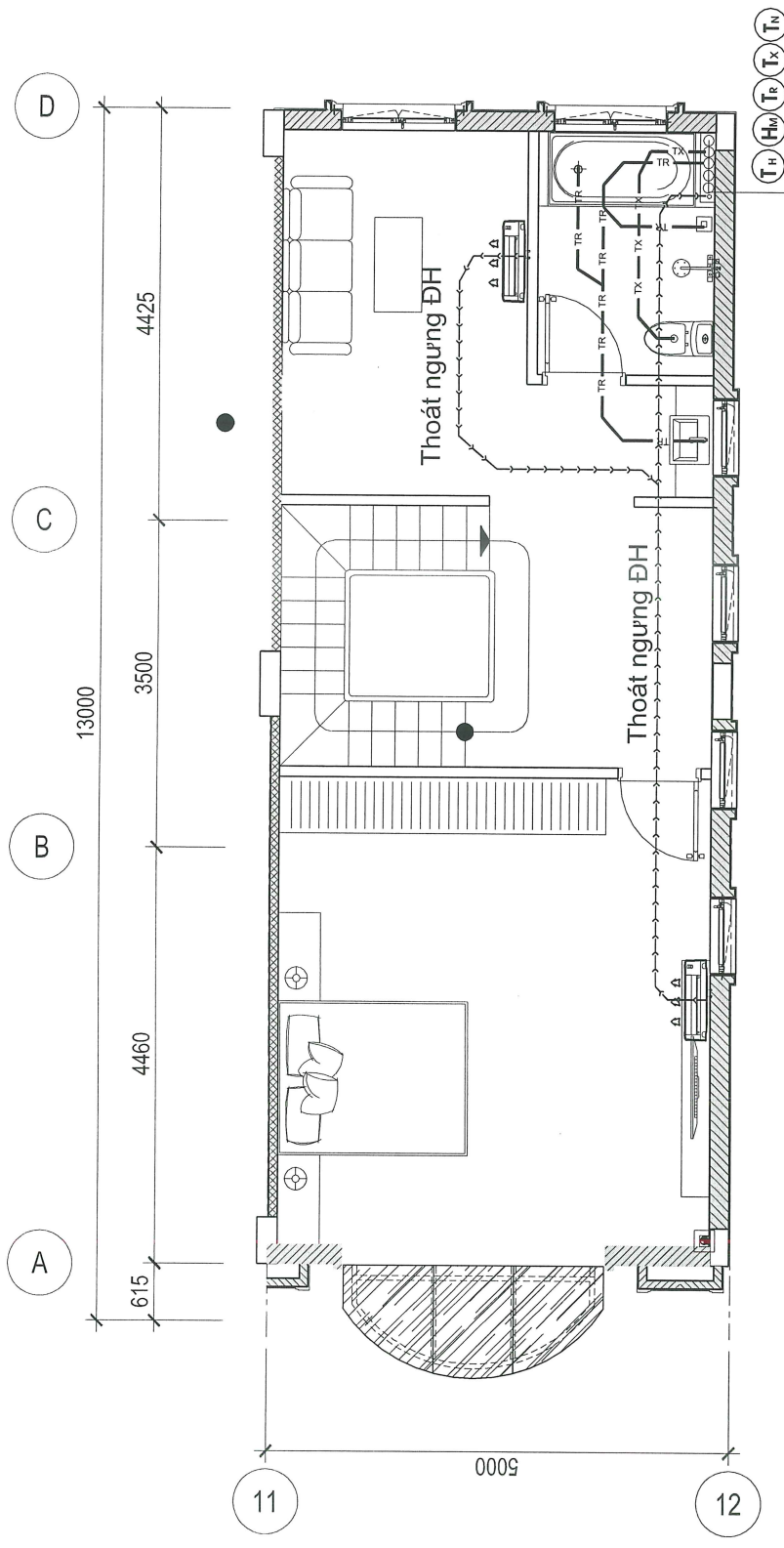
MẶT BẰNG THOÁT NƯỚC TẦNG 2
