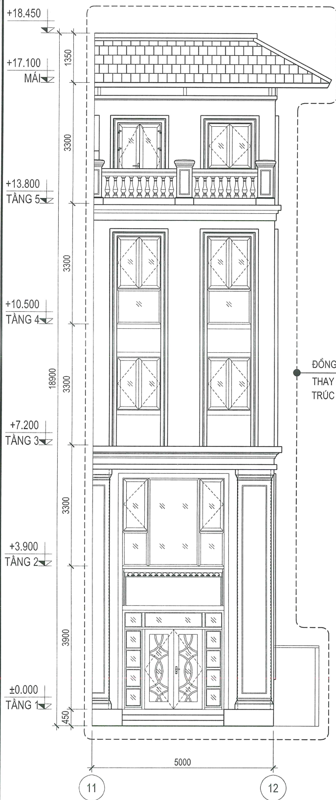
MẶT ĐỪNG HIỆN TRẠNG TRỤC 11-12
