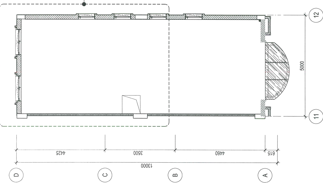
MẶT BẰNG HIỆN TRẠNG TẦNG 2
