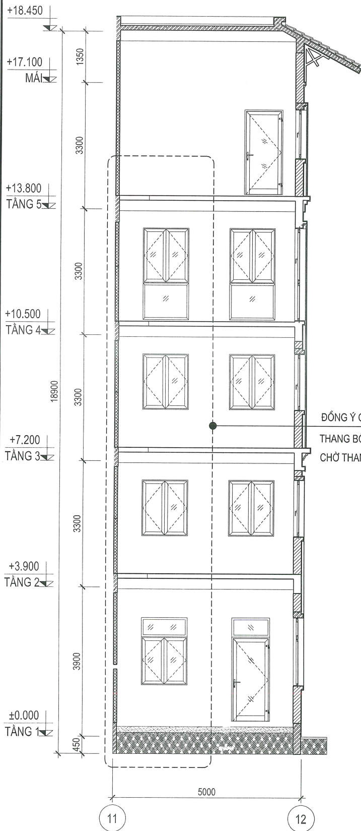
MẶT CẮT NGANG HIỆN TRẠNG
