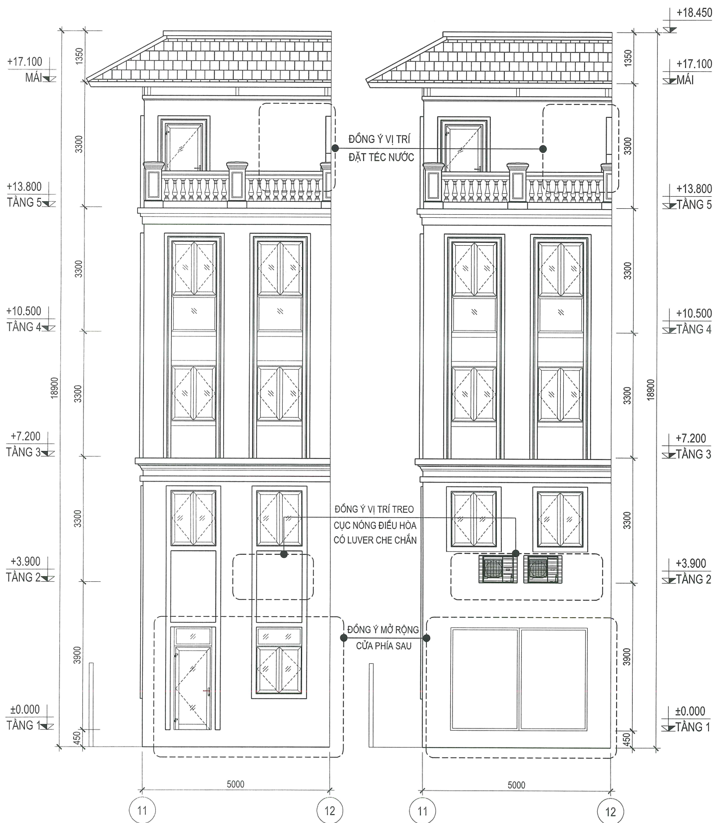
MẶT ĐỨNG HIỆN TRẠNG TRỤC 12-11
