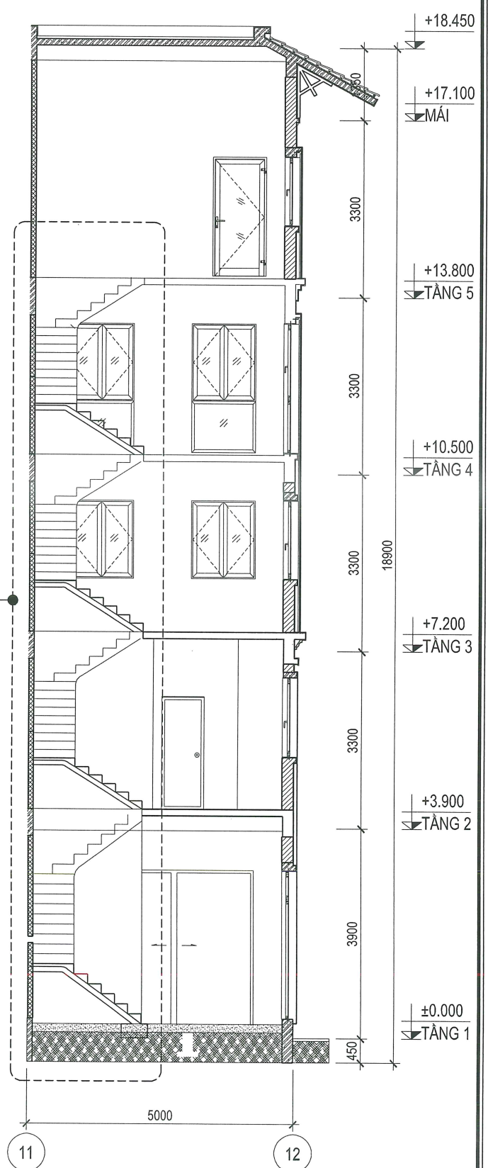
MẶT CẮT NGANG CẢI TẠO
