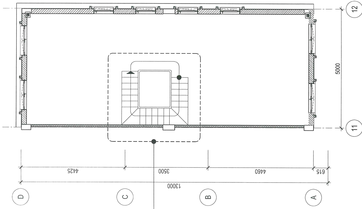
MẶT BẰNG CẢI TẠO TẦNG 3
