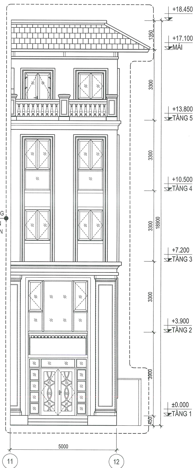
MẶT ĐỪNG CẢI TẠO TRỤC 11-12
