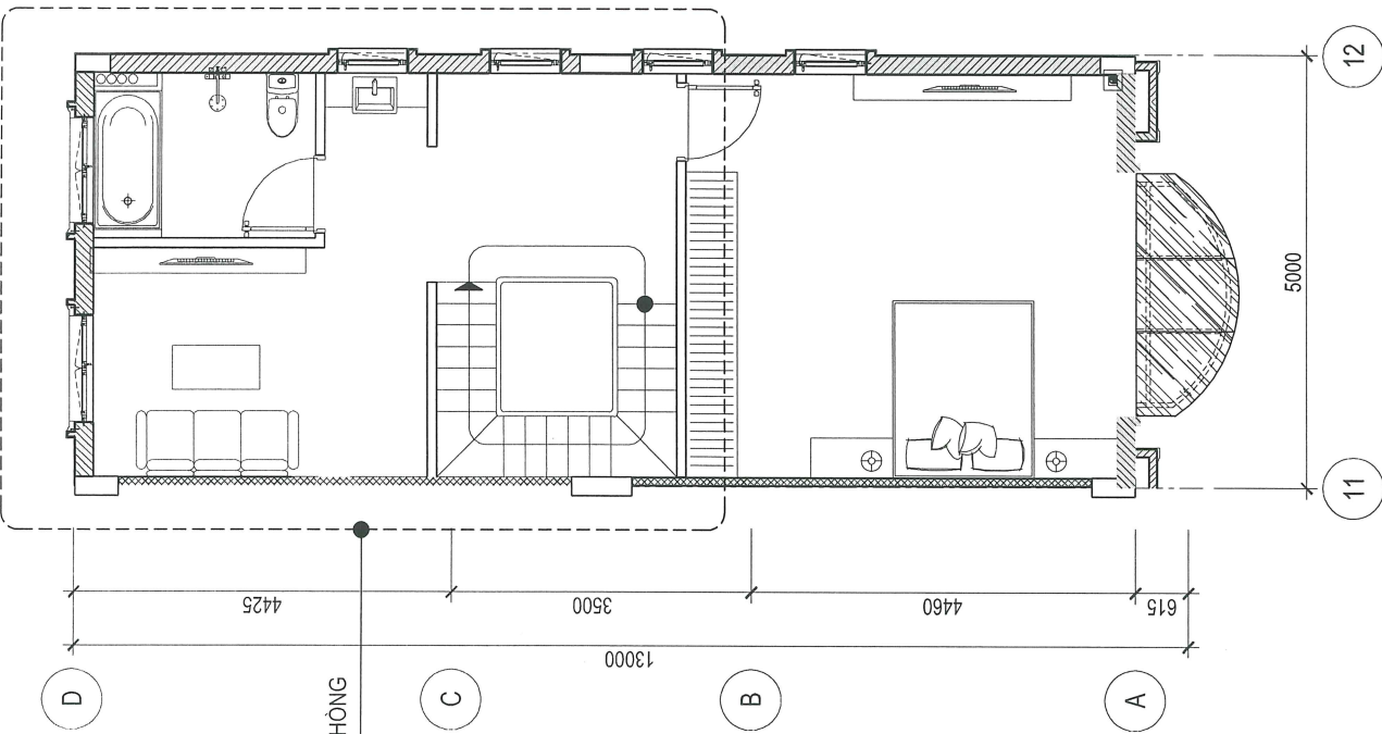
MẶT BẰNG CẢI TẠO TẦNG 2
