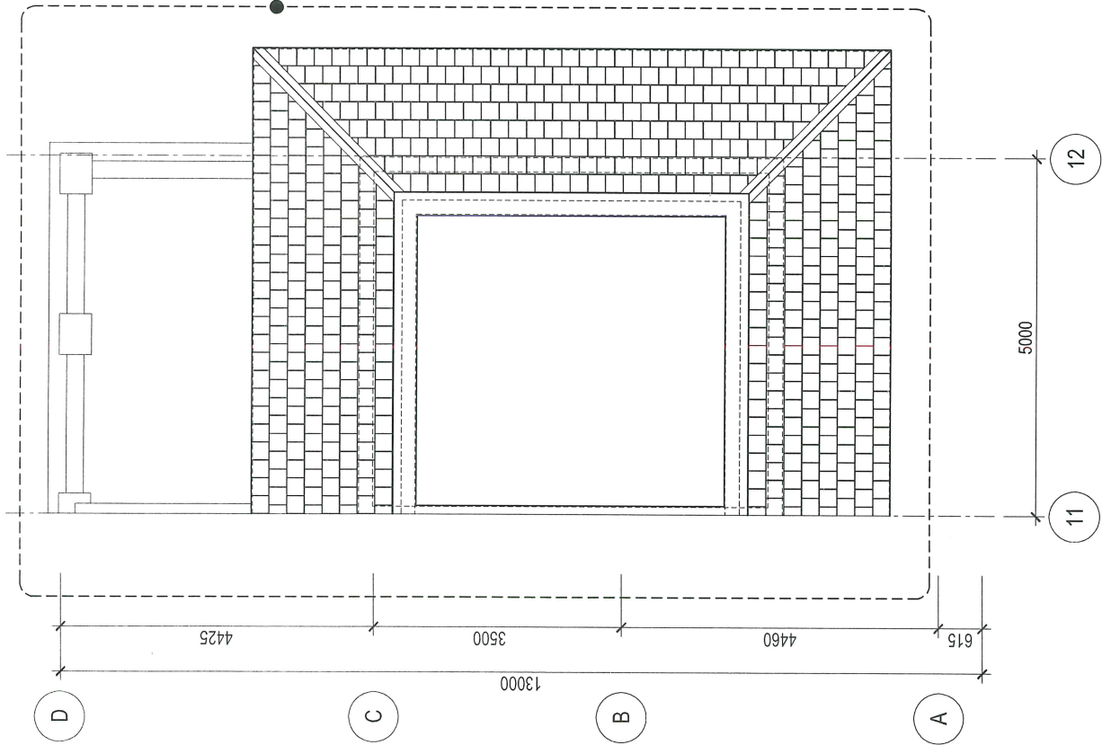
MẶT BẰNG HIỆN TRẠNG Mái
